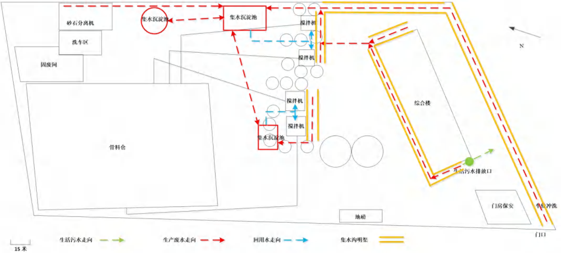
附图 11 项目废水走向图
