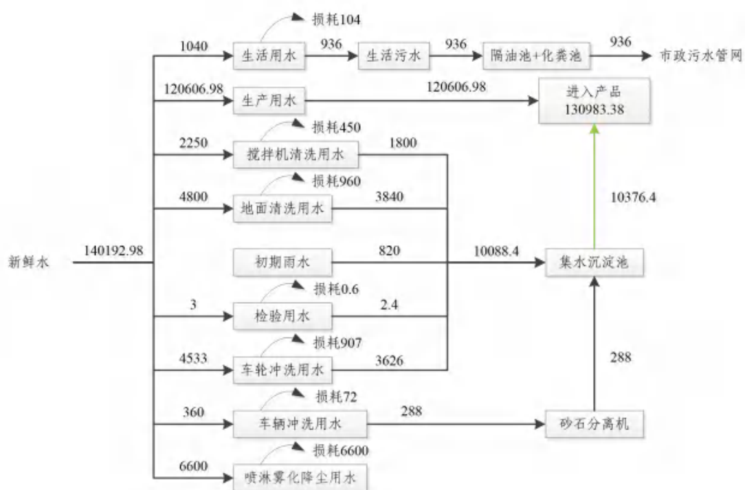
图 2-3 项目扩建后水平衡图 单位：m³/a
