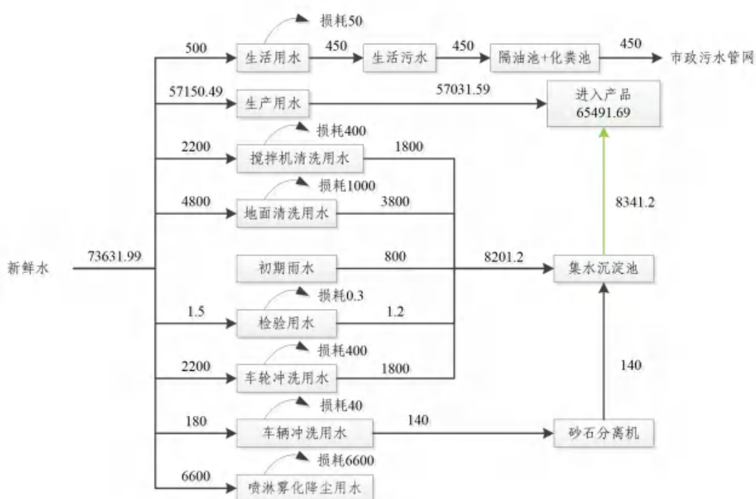
图 2-2 现有项目水平衡图 单位： \text{m}^3/\text{a}
