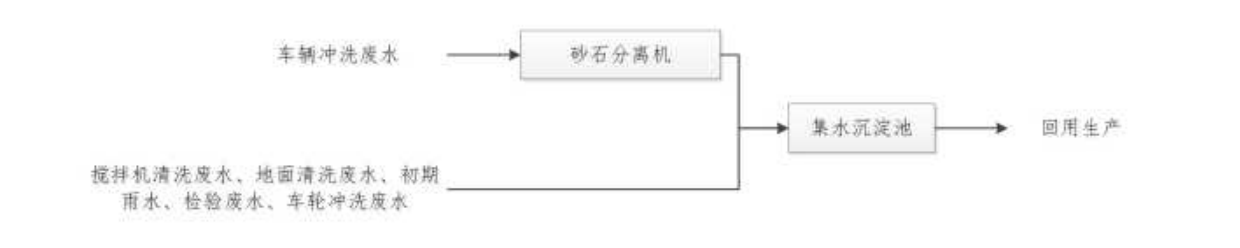
图 4-1 生产废水、初期雨水处理工艺流程图
