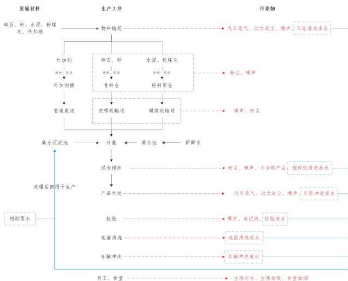
图2-5 项目生产工艺流程图
