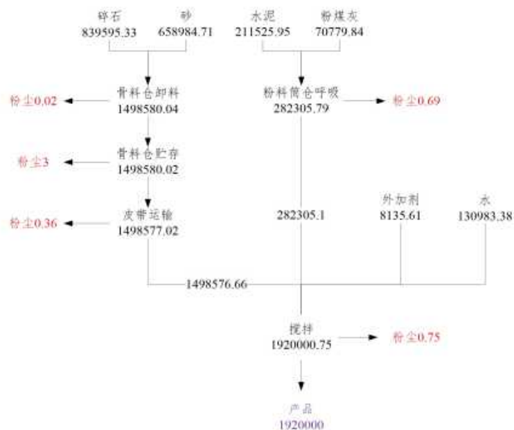
图2-3 项目扩建后物料平衡图 (单位: t/a)
