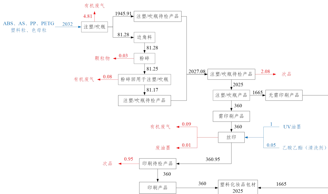
图2-3 项目物料平衡图（单位：t/a）
